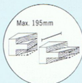
Mitred Tenon
